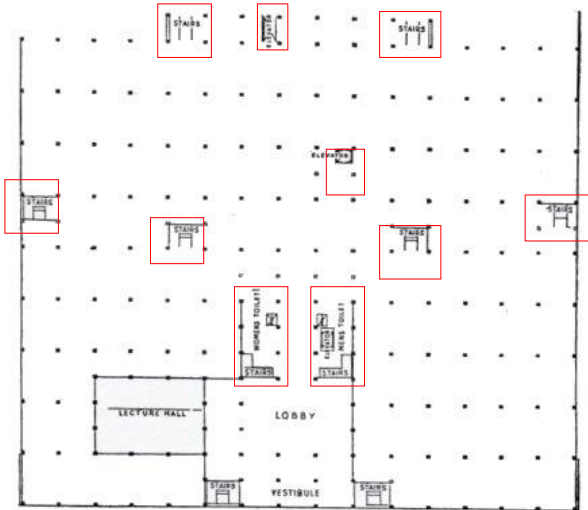
Abb. 1 Iowa City. Der Grundplan. Das leere Gebäude, wie es zur veränderbaren Einrichtung verfügbar ist. Festgelegt sind nur die eingezeichneten Gebäudeteile.
